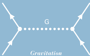
Feynman-Diagramme: Kurzschrift für Theoretiker
